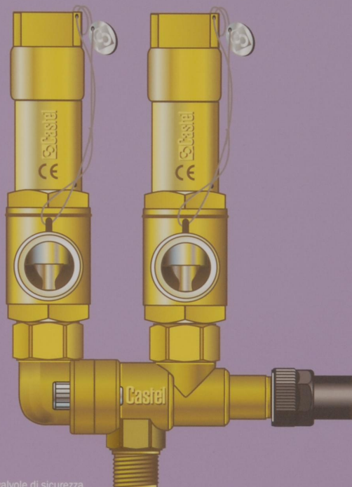
Rubinetto di servizio con coppia di valvole di sicurezza
